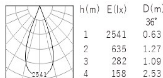
3000K 36°
