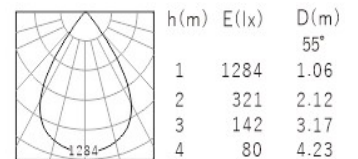
3000K 55°
